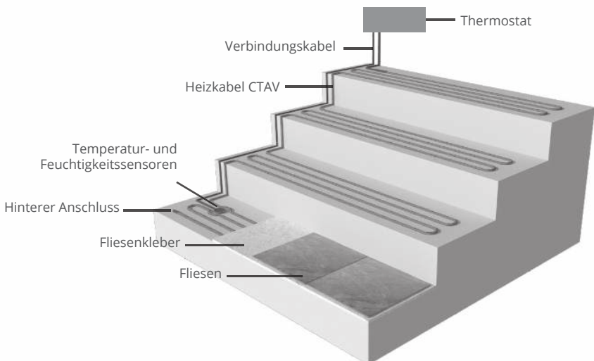
Abbildung 8. Installation von Heizkabeln an Treppen
