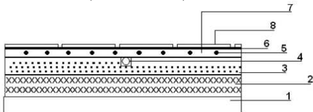
1. ábra. Új padlófűtés telepítése
